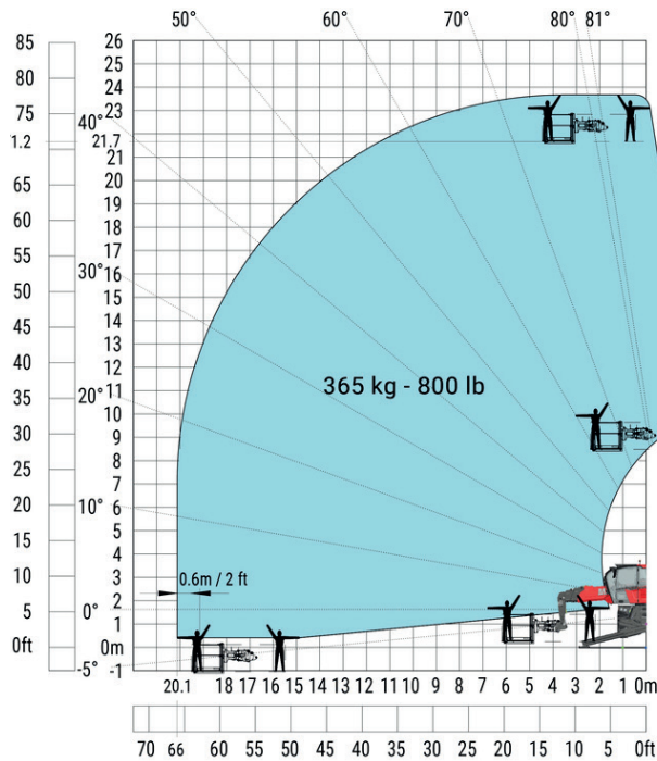
Nacelle orientable extensible 365 kg / 3 personnes
